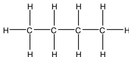
butane
